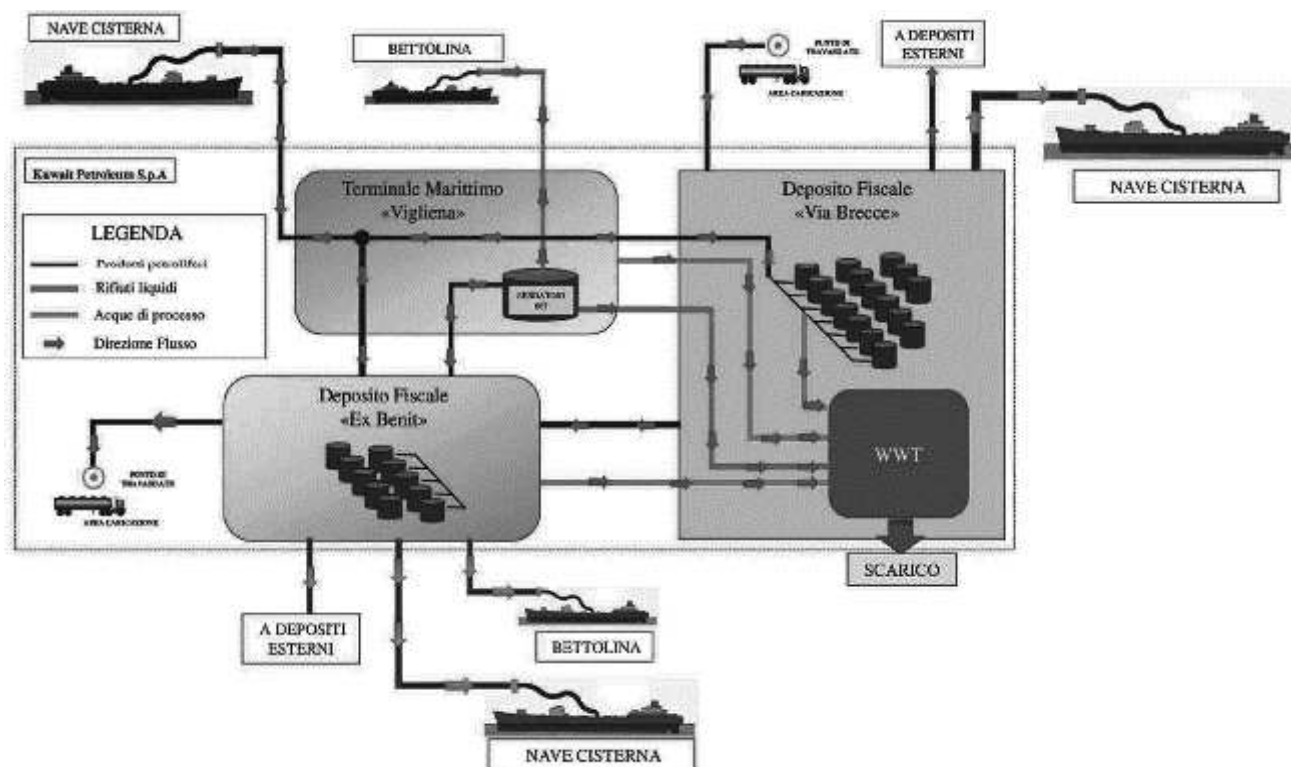
Figura 2.1: Schema semplificato delle attività produttive presso il sito della Kuwait Petroleum Italia di Napoli
